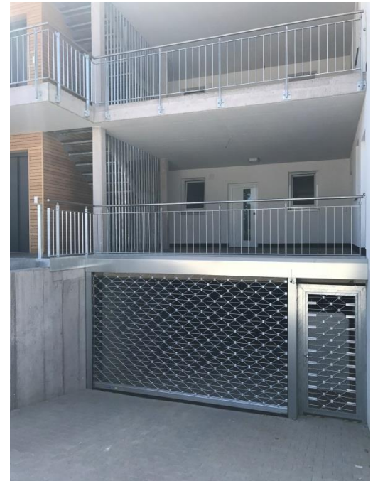
Tiefgaragen-Rollgitter MRTG plus als Vorbauelement mit Seitentüre
